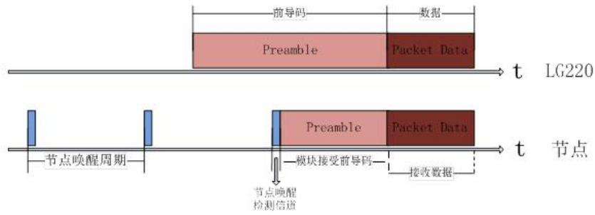
图 15 轮询唤醒模式时序
