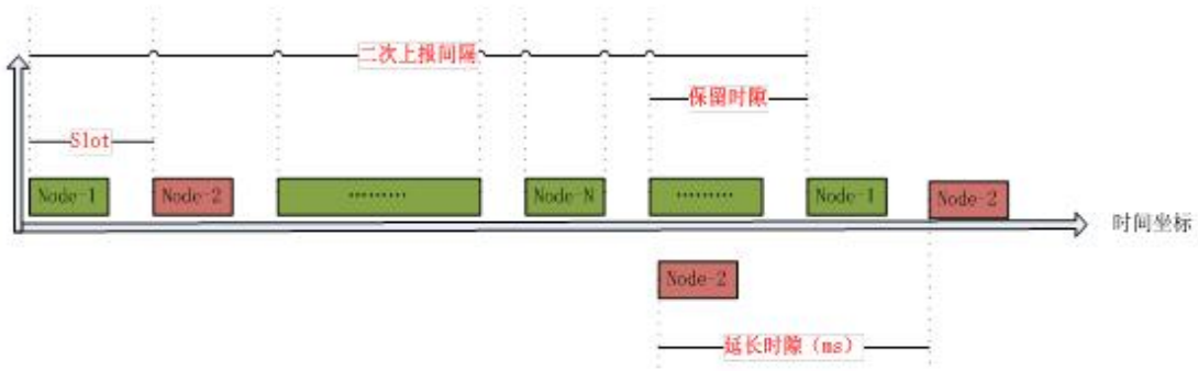
图 12 主动上报时序
