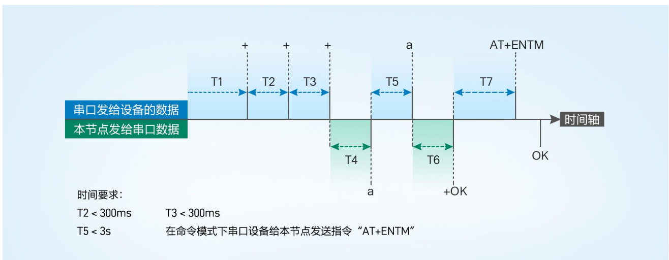
图 44 进入 AT 指令时序图
