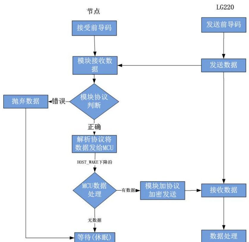
图 18 服务器主动下发简易流程
